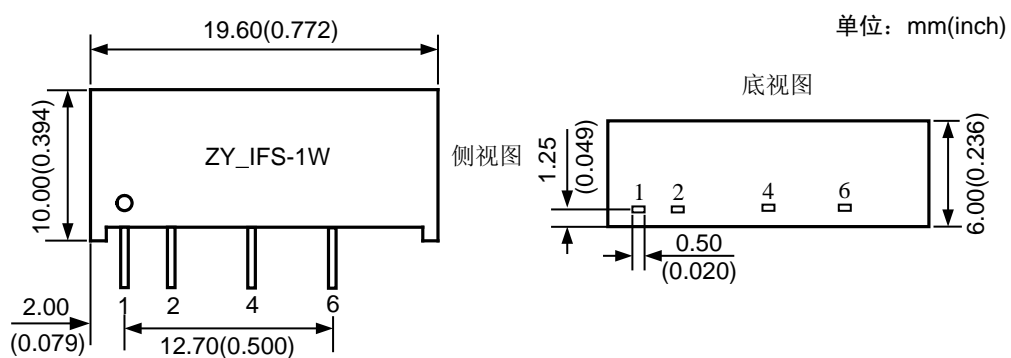
图 1.2 ZY_IFS-1W 引脚间距尺寸
