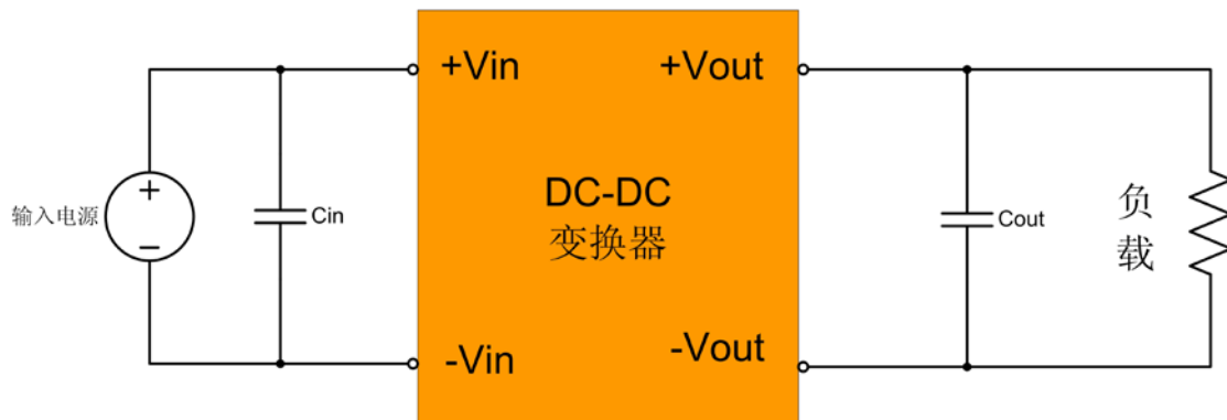
图 5.1 ZY_IFS-1W 电源模块电路连接图
