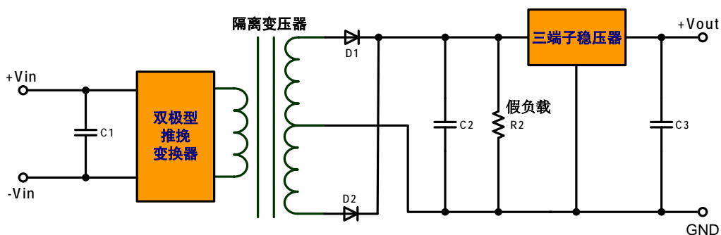
图 1 原理框图
