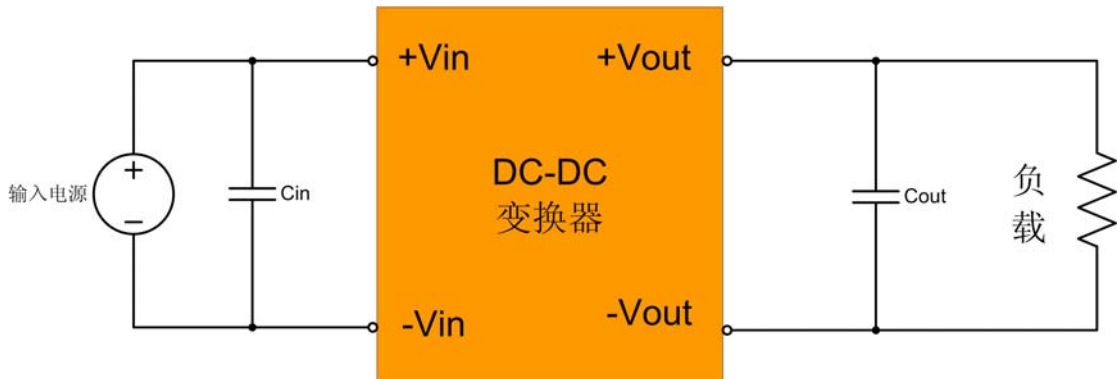
图 4.1 ZY_FKS-2W 电源模块电路连接图
