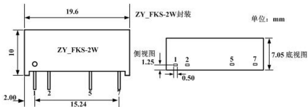
图 2.1 ZY_FKS-2W 引脚尺寸
