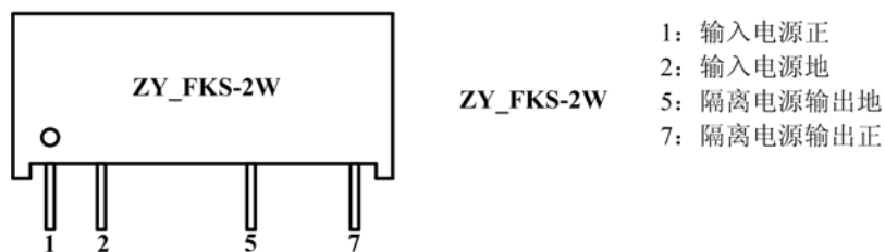
图 1.2 引脚分布图
