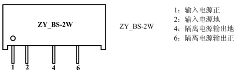
图 1.2 引脚分布图
