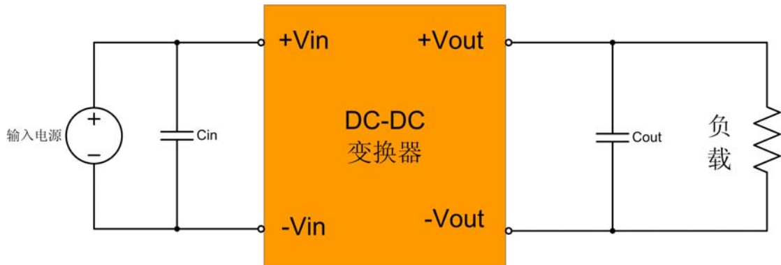
图 4.1 ZY_BS-2W 电源模块电路连接图
