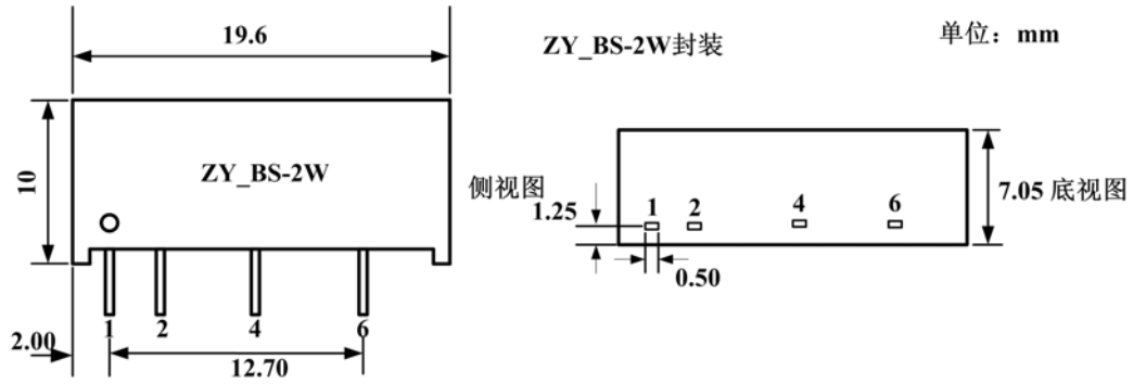
图 2.1 ZY_BS-2W 外观机械尺寸
