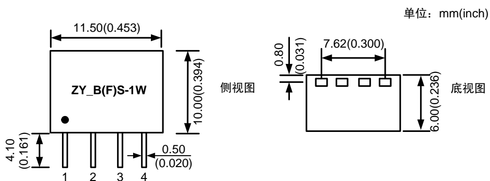
图 1.2 ZY_B(F)S-1W 引脚尺寸
