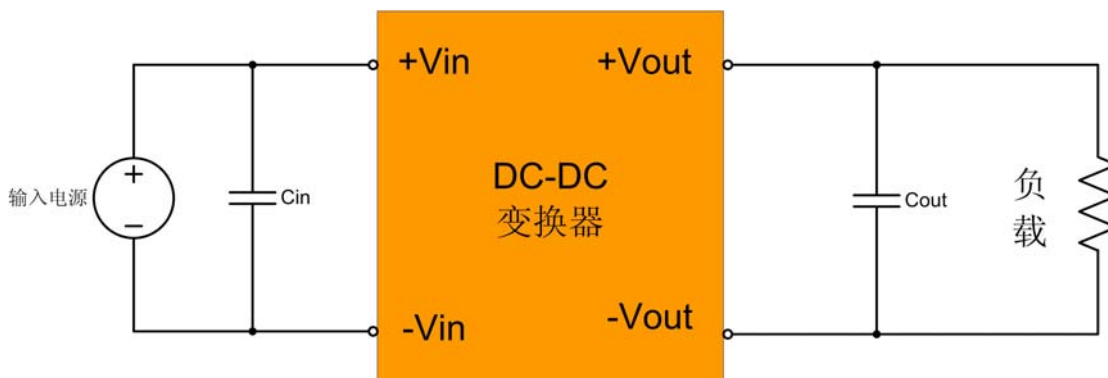
图 4.1 ZY_B(F)S-1W 电源模块电路连接图
