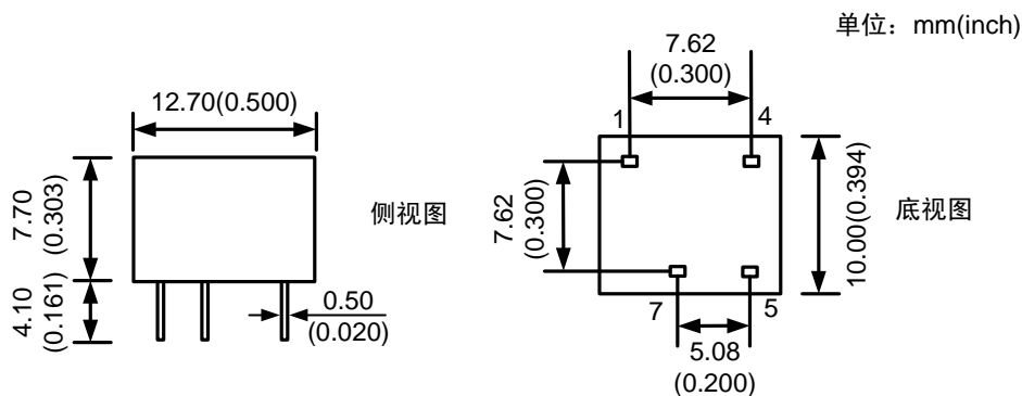
图 1.3 ZY_B(F)D-1W 引脚尺寸
