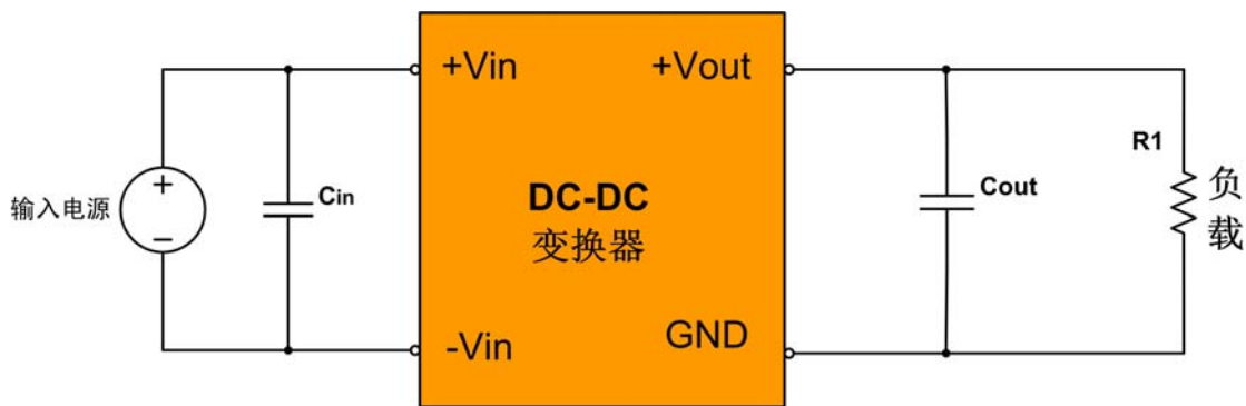
图 5.1 ZY_B(F)D-1W 接口电路
