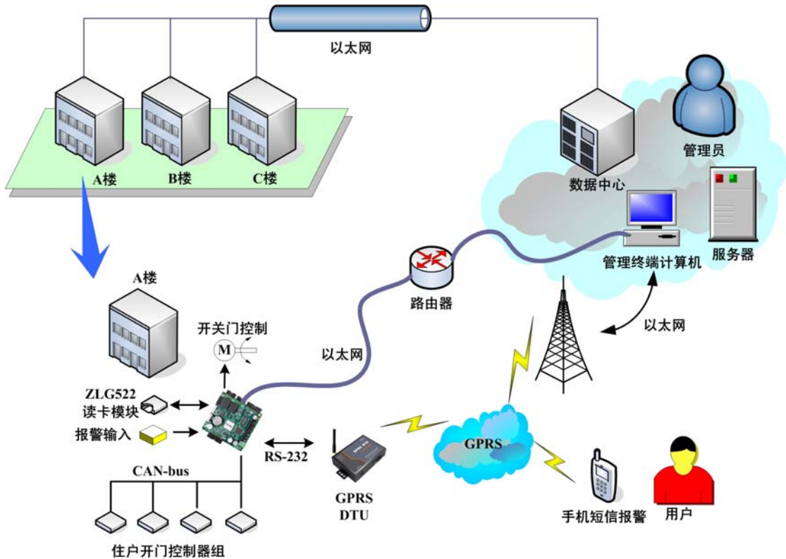
图 2 智能小区门禁系统解决方案示意图
