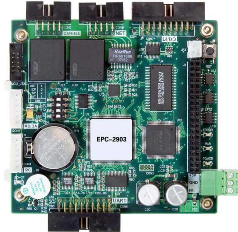
图 1 EPC2000 产品实物图
