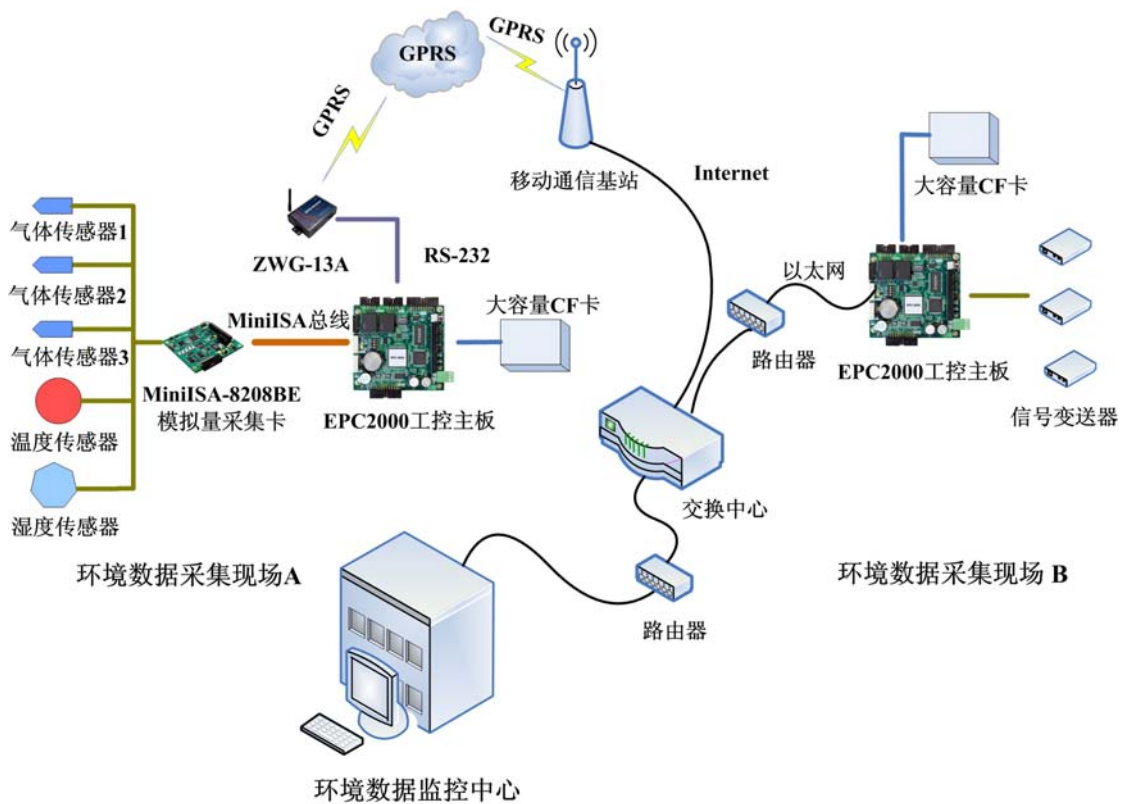
图 2.1 环境监测系统应用方案
